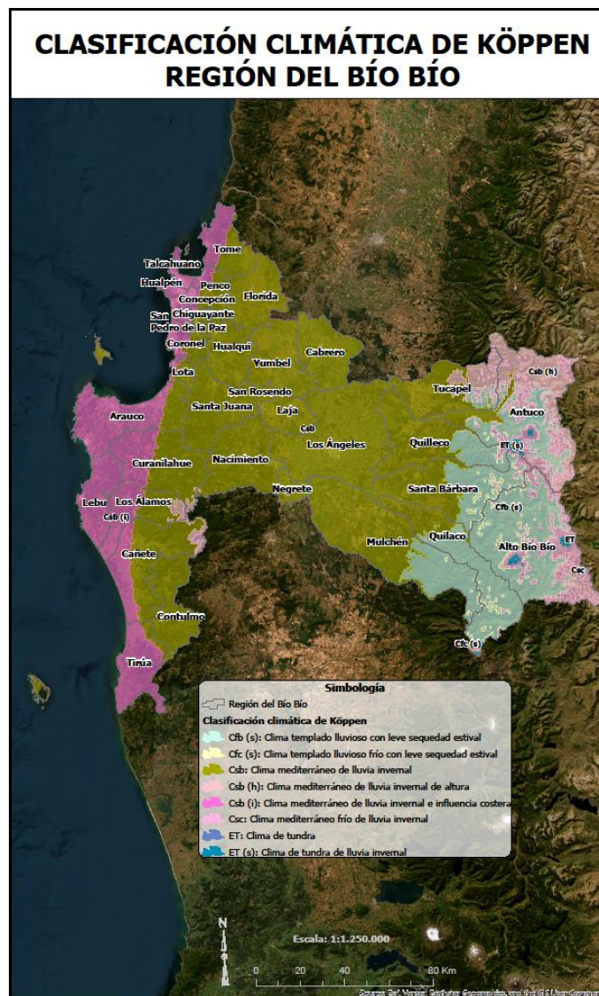
Clasificación Climática de Köppen. Región del Biobío. Fuente: Departamento de Geografía Universidad de Chile, 2017.
