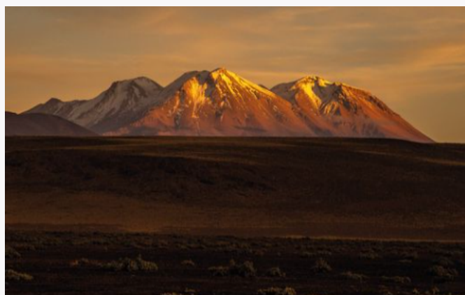
Volcán Aucanquilcha
